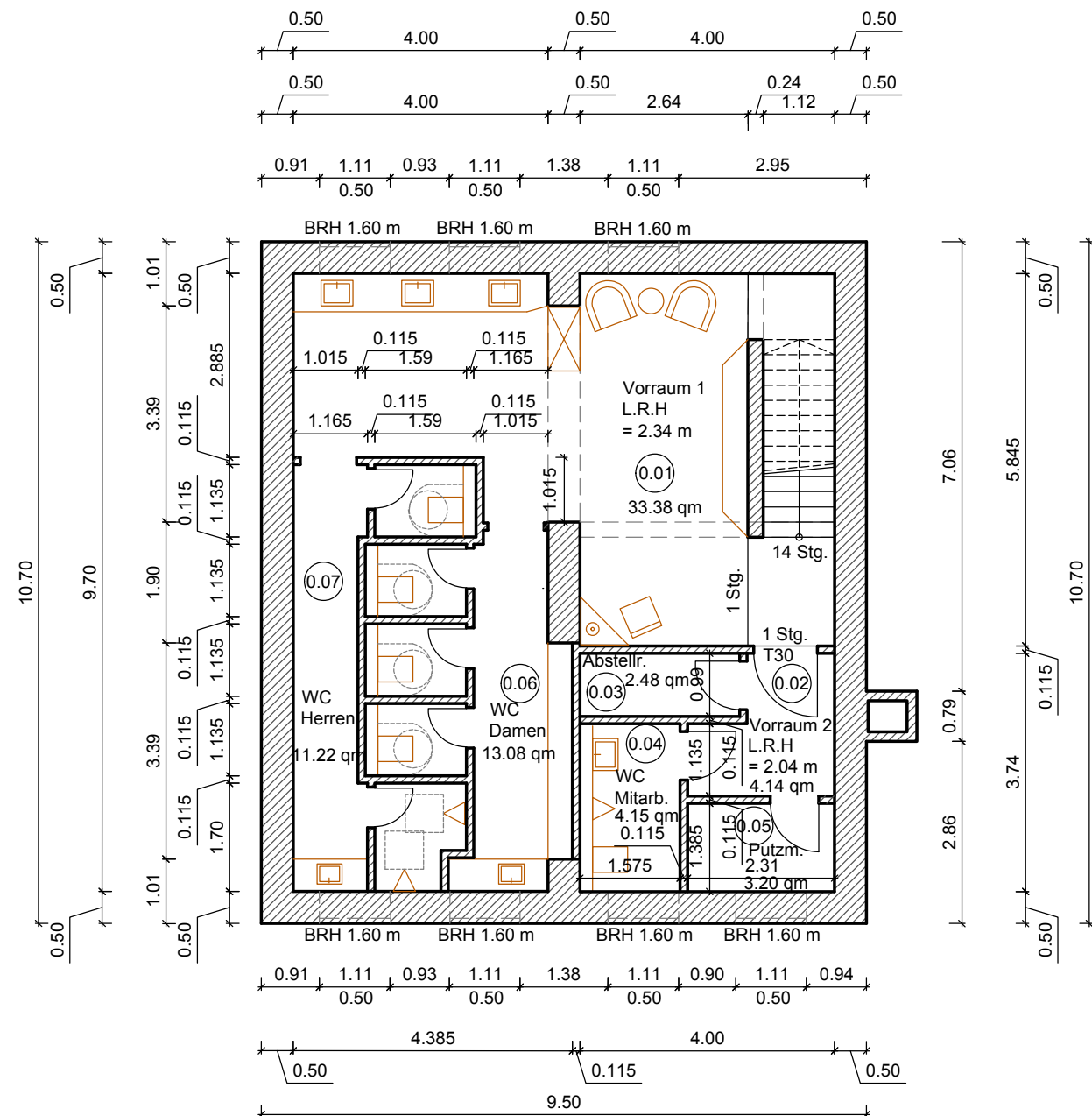
Kellergrundriss
